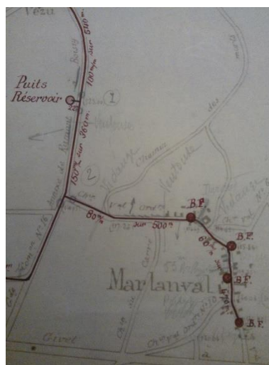
Plan général des canalisations où l'on retrouve la localisation des 13 bornes fontaines et d'incendie dans les trois hameaux.
